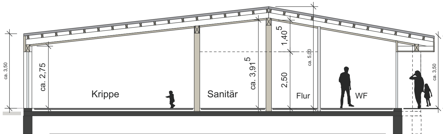
Schnitt A-A
